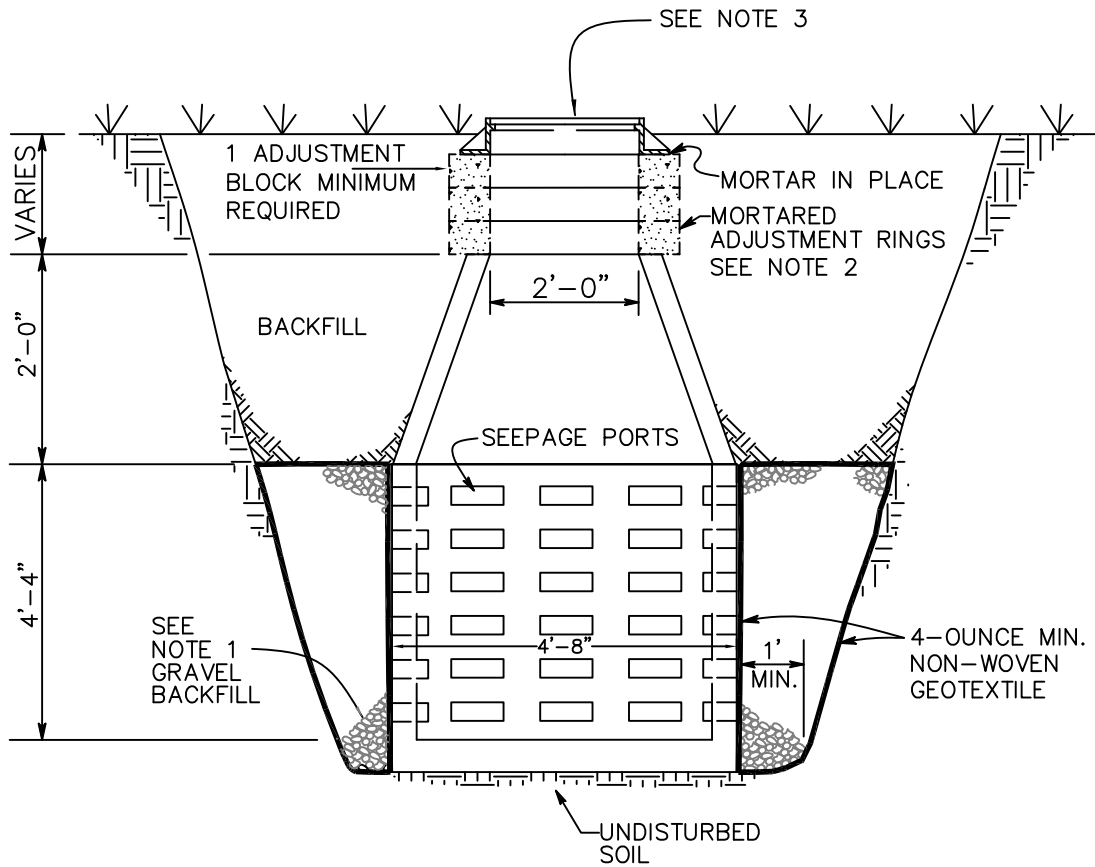
DRYWELL - TYPE 'A'
